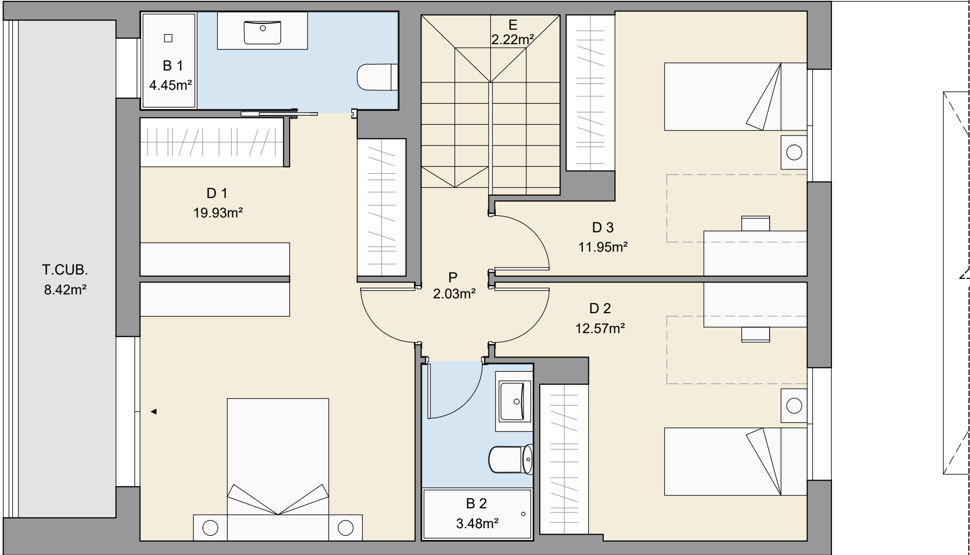
PLANTA PRIMERA
