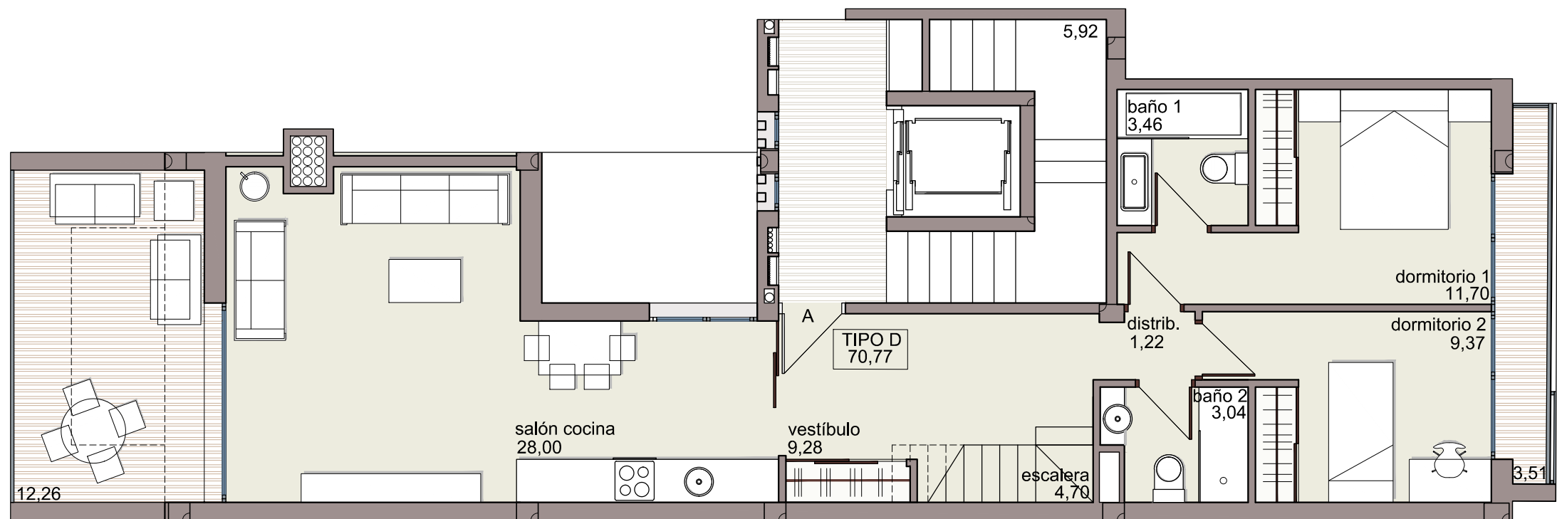
PLANTA CUARTA
