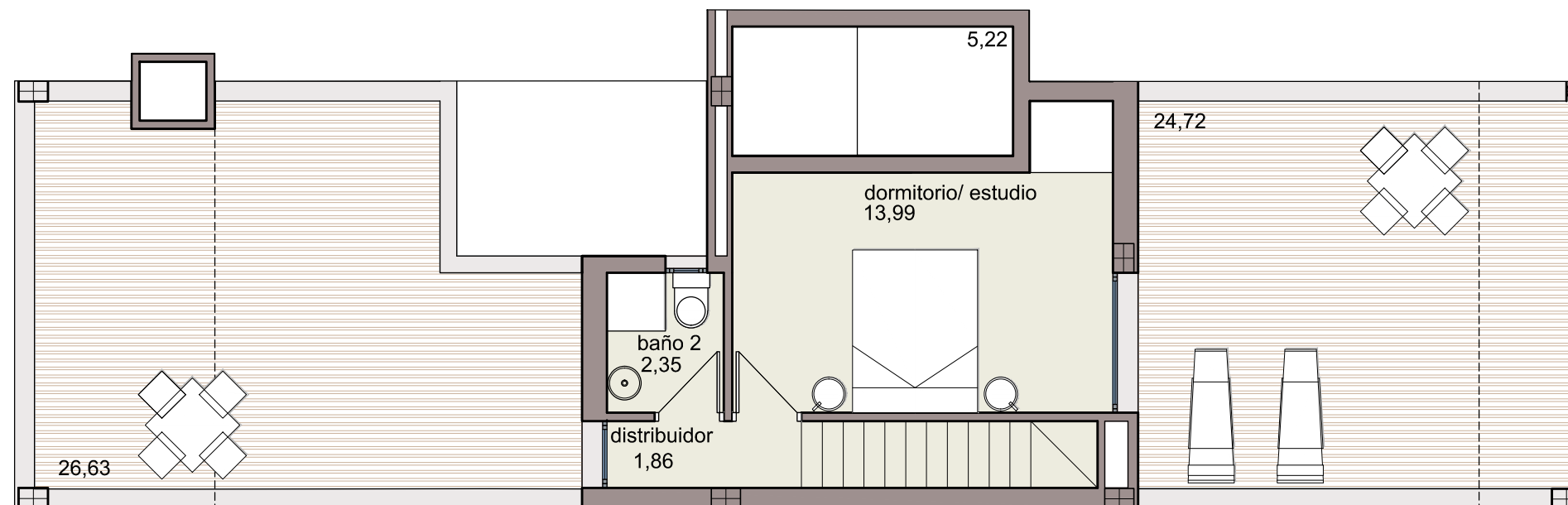
PLANTA BAJO CUBIERTA
